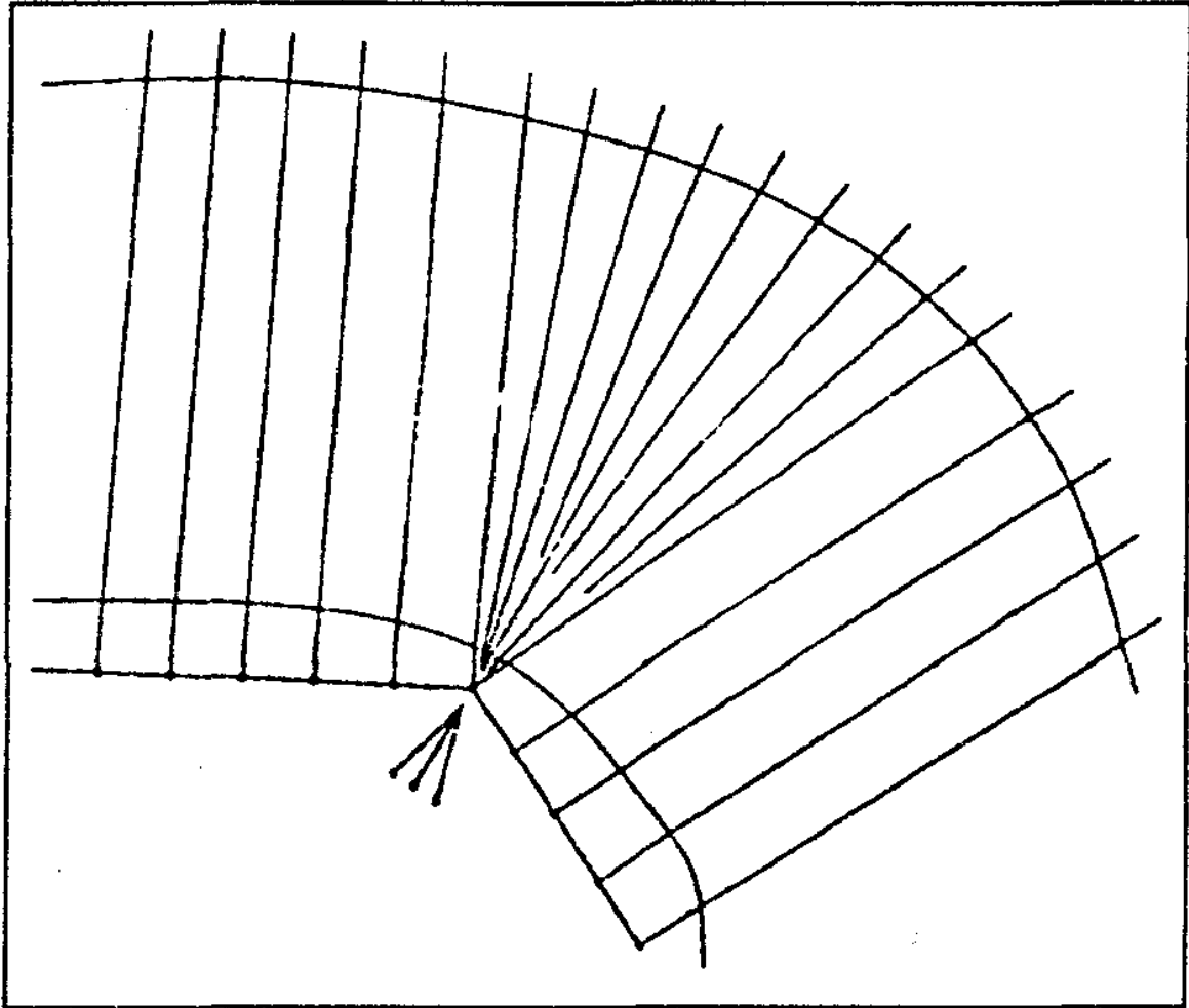
Рис. 1. Схема разбивки радиальных галсов
