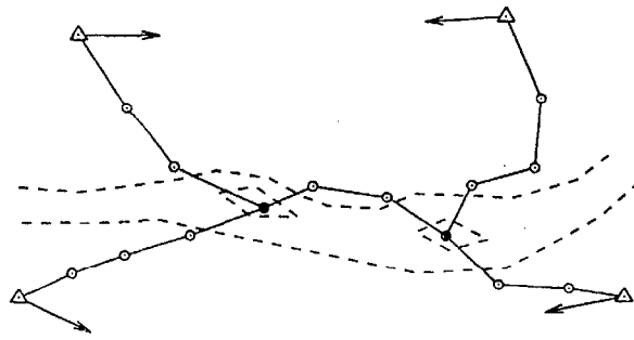
3. Схема полигонометрических ходов с двумя узловыми точками
