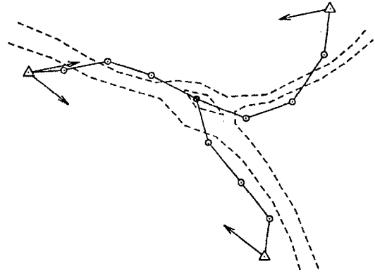
2. Схема полигонометрических ходов с одной узловой точкой
