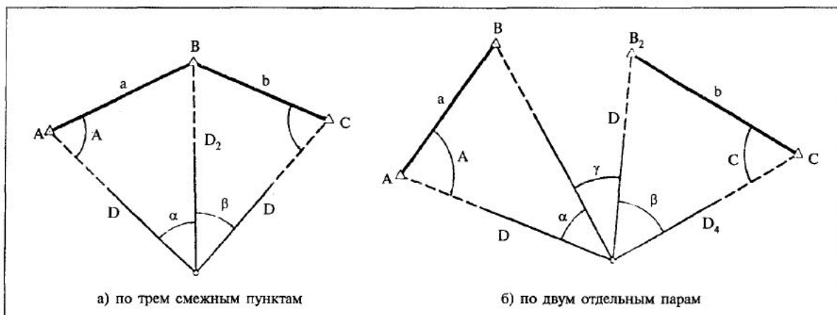
Рис. 2. Схема определения места на галсе двумя секстанами.
