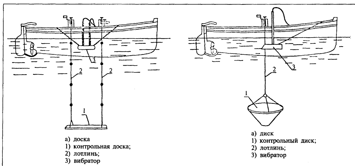
Рис. 3. Тарирующие устройства эхолота
